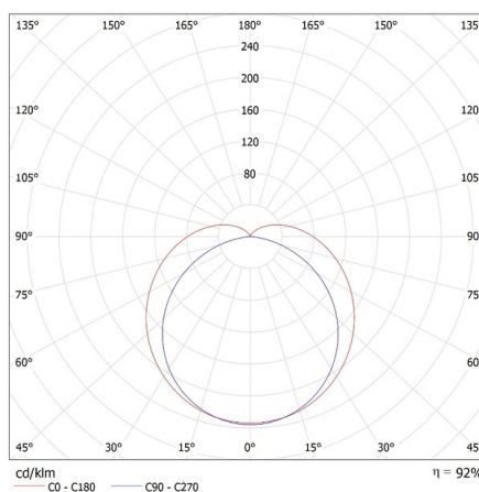
KANLUX S.A. (kat 38942) TP SLIM TW N 40W-NW / Krzywa rozsyłu światła (biegunowo)
