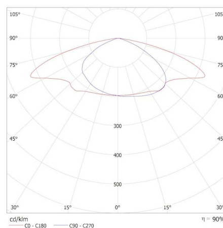
KANLUX S.A. (kat 39300) PRO-S S 65W-ZH NW / Krzywa rozsyłu światła (biegunowo)
