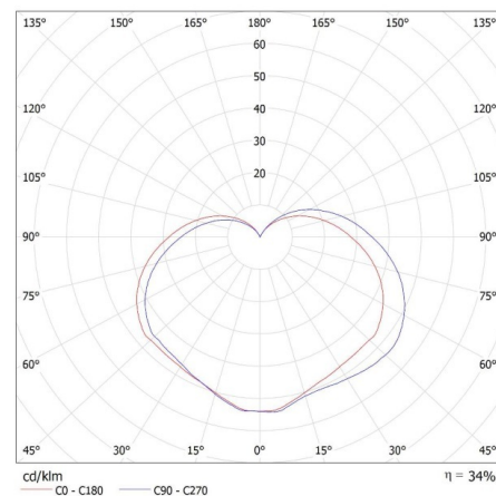
KANLUX S.A. (kat 36548) LAVEN EL 25 GR + IQ-LED / LDC (Polar)
