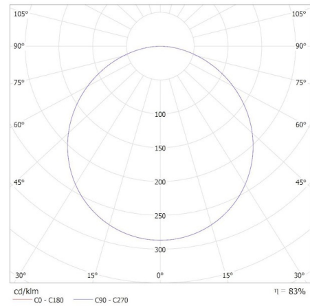
KANLUX S.A. (kat 37176) BLINGO 38W 4560 60NW / Krzywa rozsytu światła (biegunowo)
