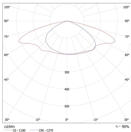
KANLUX S.A. (kat 39292) PRO-S S 25W-ZH NW / Krzywa rozsytu światła (biegunowo)
