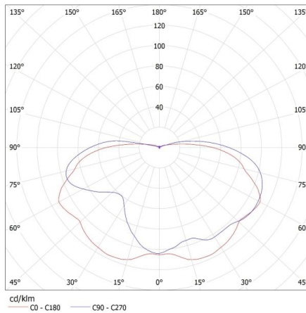
KANLUX S.A. (kat 70523) MILO 7040T P / Krzywa rozsyłu światła (biegunowo)
