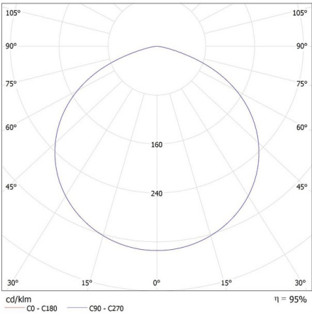
KANLUX S.A. (kat 27158 + 38139 + 38135) HB PRO STRONG 150W-NW + LENS 120D + GRID / Krzywa rozsyłu światła (biegunowo)
