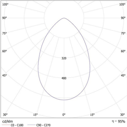
KANLUX S.A. (kat 27158 + 38138 + 38135) HB PRO STRONG 150W-NW + LENS 60D + GRID / Krzywa rozsyłu światła (biegunowo)
