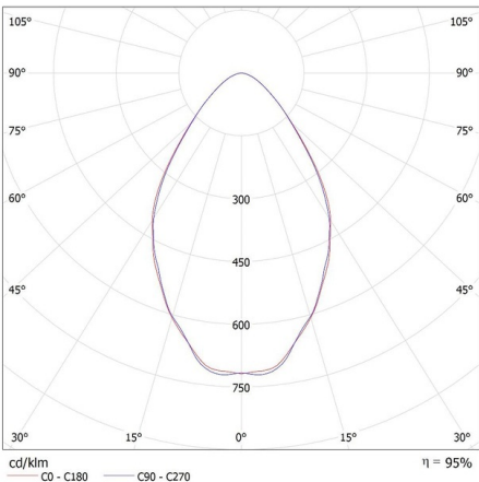
KANLUX S.A. (kat 27159 + 38128 + 38136) HB PRO STRONG 200W-NW + LENS 60D + GRID / Krzywa rozsyłu światła (biegunowo)
