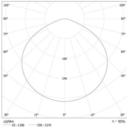
KANLUX S.A. (kat 27159 + 38129 + 38136) HB PRO STRONG 200W-NW + LENS 120D + GRID / Krzywa rozsyłu światła (biegunowo)
