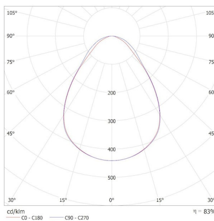
KANLUX S.A. (kat 37265) BLINGO U E125LM 60NW / Krzywa rozsyłu światła (biegunowo)
