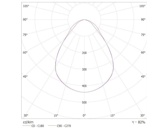
KANLUX S.A. (kat 37278) BLINGO U29-35W 120CCT 3000K / Krzywa rozsyłu światła (biegunowo)
