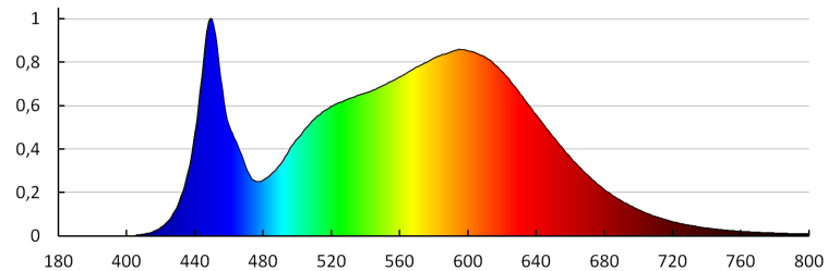
KANLUX S.A. (kat 22609) MAH LED HI 26W-NW RYF / LDC (Polar)
