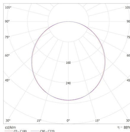
Miledo (kat 31129) BAREV 2X36W3600 120NW / Krzywa rozsytu światła (biegunowo)
