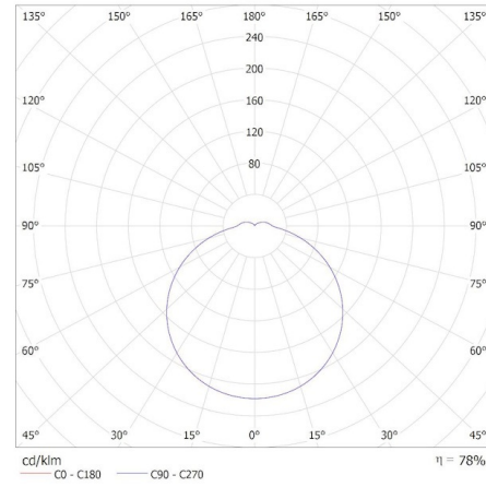
KANLUX S.A. (kat 37296) IPER LED 26W-NW-L / Krzywa rozsywu światła (biegunowo)
