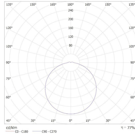
KANLUX S.A. (kat 37297) IPER LED 35W-NW-L / Krzywa rozsywu światła (biegunowo)
