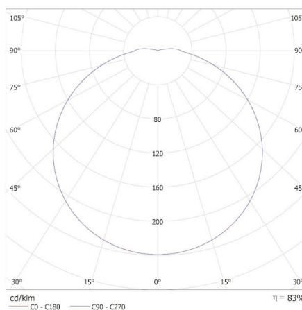
KANLUX S.A. (kat 37298) IPER LED 10W-NW-O-SE / Krzywa rozsyłu światła (biegunowo)
