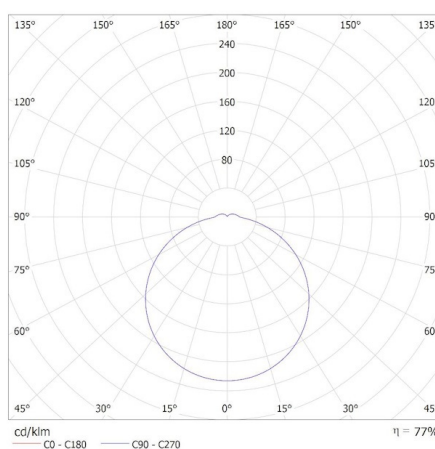
KANLUX S.A. (kat 37301) IPER LED 35W-NW-O-SE / Krzywa rozsyłu światła (biegunowo)
