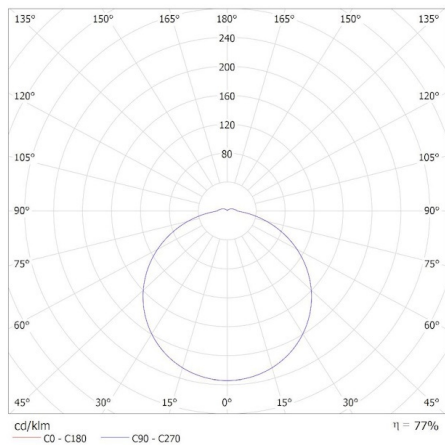
KANLUX S.A. (kat 37305) IPER LED 35W-NW-L-SE / Krzywa rozsytu światła (biegunowo)
