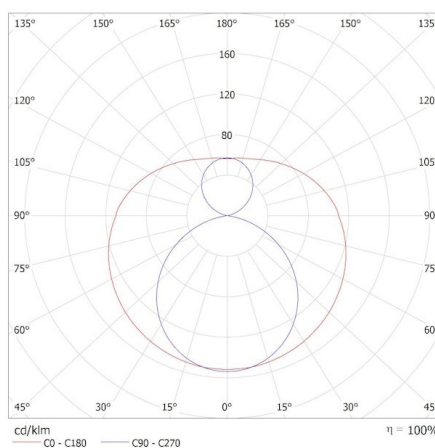
KANLUX S.A. (kat 37630) T8 LED 9-NW / Krzywa rozsyłu światła (biegunowo)
