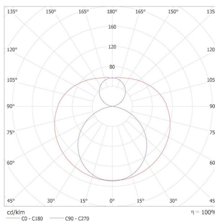
KANLUX S.A. (kat 37633) T8 LED 18-CW / Krzywa rozsyłu światła (biegunowo)
