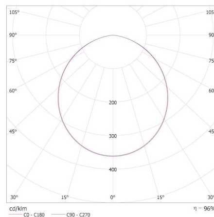
KANLUX S.A. (kat 38120) DAXA-M-IR 9W CCTDIM W / Krzywa rozsyłu światła (biegunowo)
