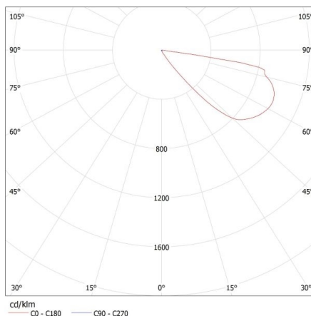
KANLUX S.A. (kat 22760) ONSTAR LED-GR / Krzywa rozsytu światła (biegunowo)
