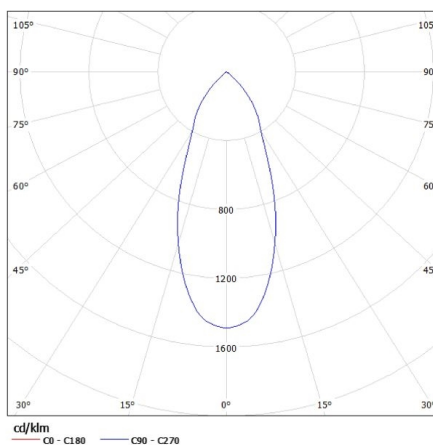
KANLUX S.A. (kat 22840) HIMA MCOB 30W / Krzywa rozsyłu światła (biegunowo)
