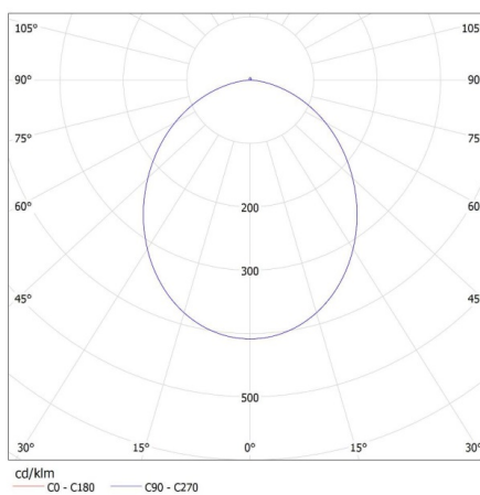
KANLUX S.A. (kat 24645) TYBIA M 25W-NW B / LDC (Polar)
