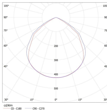
MILED o (kat 31181) GRUN V3 LED-20-B / LDC (Polar)
