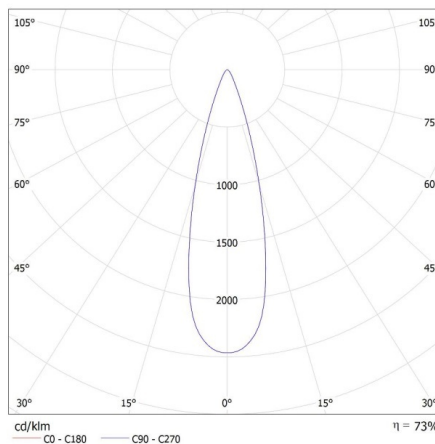
KANLUX S.A. (kat 35661) BTL 38W-940-B 15deg / LDC (Polar)
