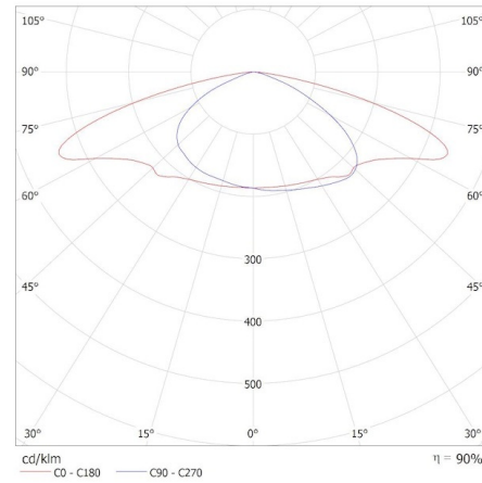
KANLUX S.A. (kat 39287) PRO-S M 105W NW / Krzywa rozsytu światła (biegunowo)
