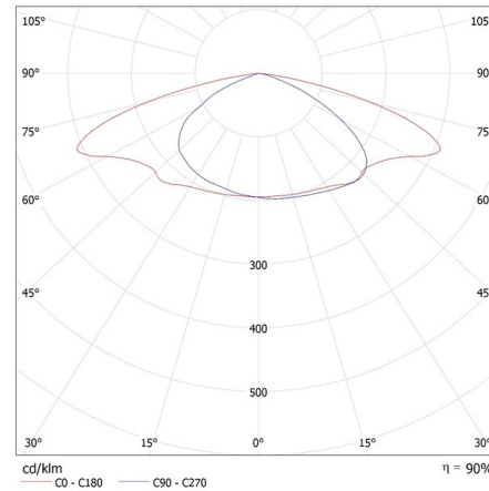
KANLUX S.A. (kat 39296) PRO-S S 45W-ZH NW / Krzywa rozsytu światła (biegunowo)
