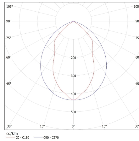
MILEDO (kat 31059) RSTR N 418/4LED/PT-H i T8 Miledo / LDC (Polar)
