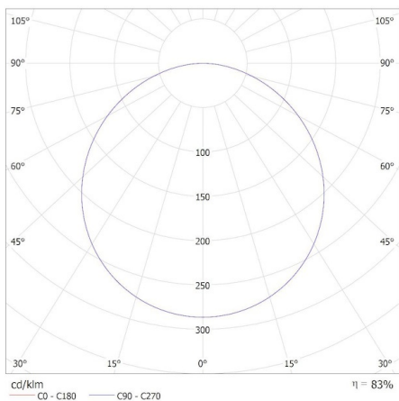
KANLUX S.A. (kat 33177) BLINGO TN 38W 6060 NW / Krzywa rozsytu światła (biegunowo)
