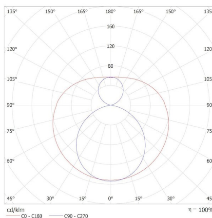
KANLUX S.A. (kat 37631) T8 LED 9-CW / Krzywa rozsyłu światła (biegunowo)
