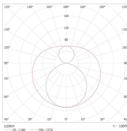
KANLUX S.A. (kat 37635) T8 LED 22-CW / Krzywa rozsyłu światła (biegunowo)
