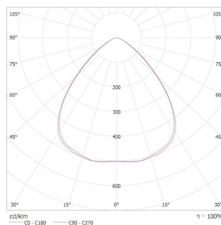
KANLUX S.A. (kat 38415) XLED GU10 6,5W-CW / Krzywa rozsyłu światła (biegunowo)
