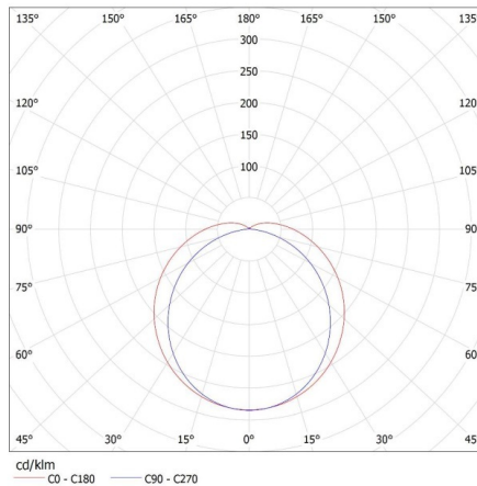
KANLUX S.A. (kat 22605) MAH-LED N 50W-NW / Krzywa rozsytu światła (biegunowo)
