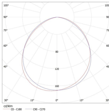
KANLUX S.A. (kat 23123) JASMIN 270-W + IQ-LED / LDC (Polar)
