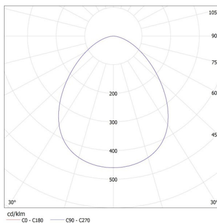
KANLUX S.A. (kat 25781) IVIAN LED 4,5W SN-WW / Krzywa rozsytu światła (biegunowo)
