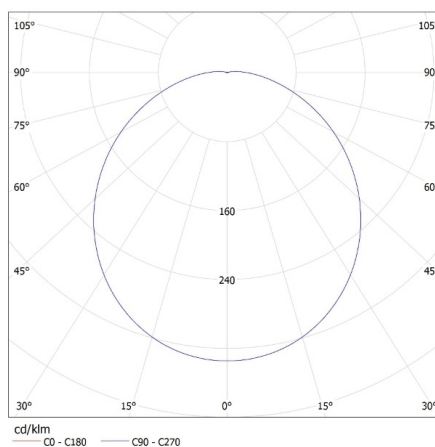
KANLUX S.A. (kat 29161) ORTE LED 24W-NW-O / LDC (Polar)
