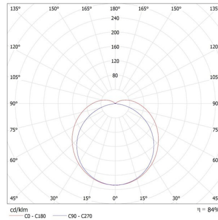
MILED o (kat 31410) DIGHT LED 18W-NW / LDC (Polar)
