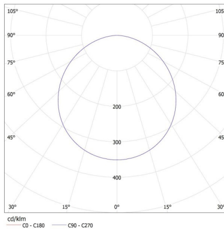
KANLUX S.A. (kat 33546) KANTI V2LED 6W-NW-W / LDC (Polar)
