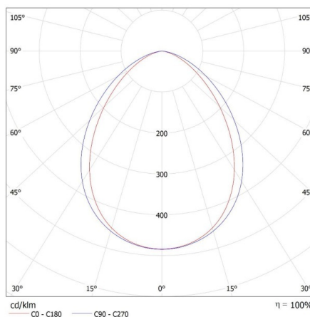
KANLUX S.A. (kat 33880) IQ-LED FL-10W-NW / LDC (Polar)
