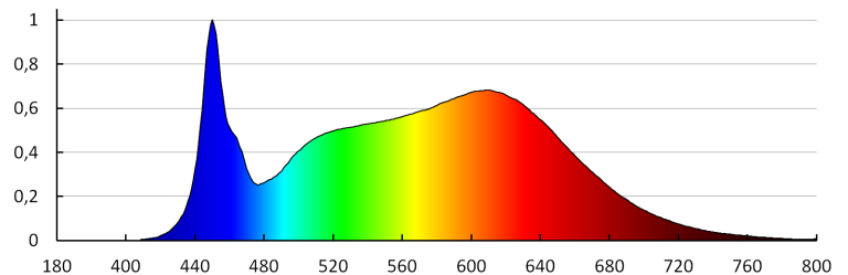
KANLUX S.A. (kat 35677) TIBERI PRO NT20W-940B / LDC (Polar)
