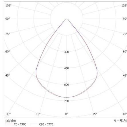
KANLUX S.A. (kat 35858) OS-S8D-NW-RST-W-N1 / Krzywa rozsyłu światła (biegunowo)
