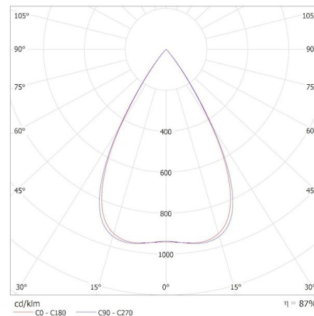
KANLUX S.A. (kat 37108) HR-SL-WW-W-RM / Krzywa rozsyłu światła (biegunowo)
