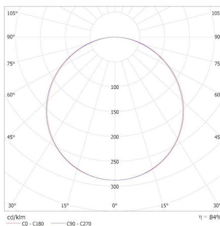
KANLUX S.A. (kat 39236) BLINGO AIO RM38W 120 / Krzywa rozsyłu światła (biegunowo)
