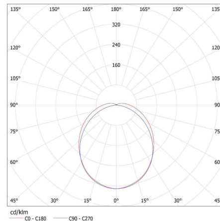
KANLUX S.A. (kat 28631) FT1200 37W-840-RYF / LDC (Polar)
