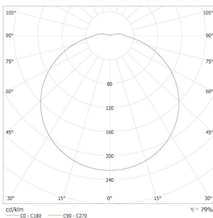
KANLUX S.A. (kat 37295) IPER LED 19W-NW-L / Krzywa rozsytu światła (biegunowo)
