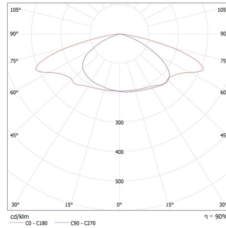
KANLUX S.A. (kat 39290) PRO-S S 15W-ZH NW / Krzywa rozsytu światła (biegunowo)
