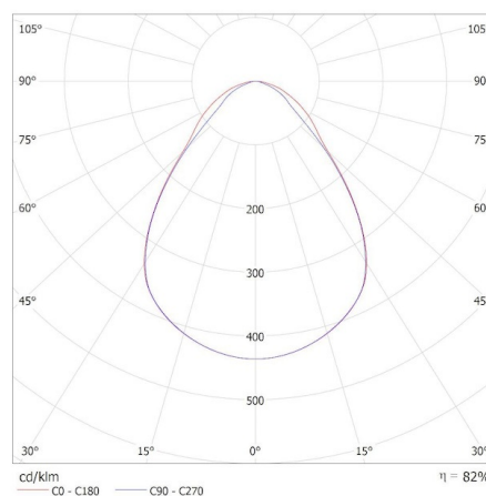
KANLUX S.A. (kat 37173) BLINGO U34W 4080 60NW / Krzywa rozsytu światła (biegunowo)
