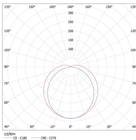
KANLUX S.A. (kat 22604) MAH-LED N 40W-NW / Krzywa rozsyłu światła (biegunowo)
