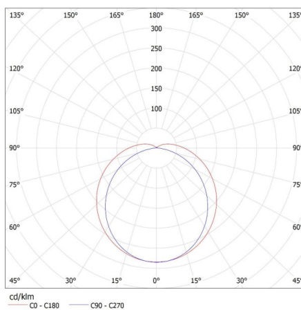
KANLUX S.A. (kat 22605) MAH-LED N 50W-NW / Krzywa rozsyłu światła (biegunowo)
