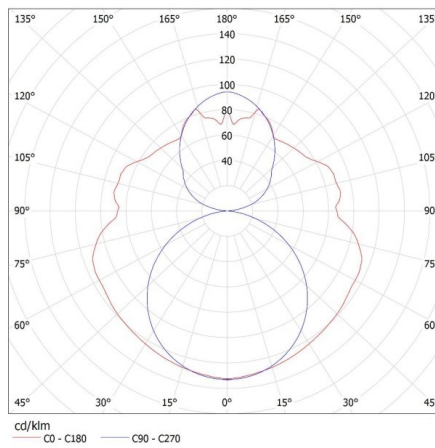
KANLUX S.A. (kat 26365) ALDO 4LED 2X150 + Miledo / Krzywa rozsytu światła (biegunowo)
